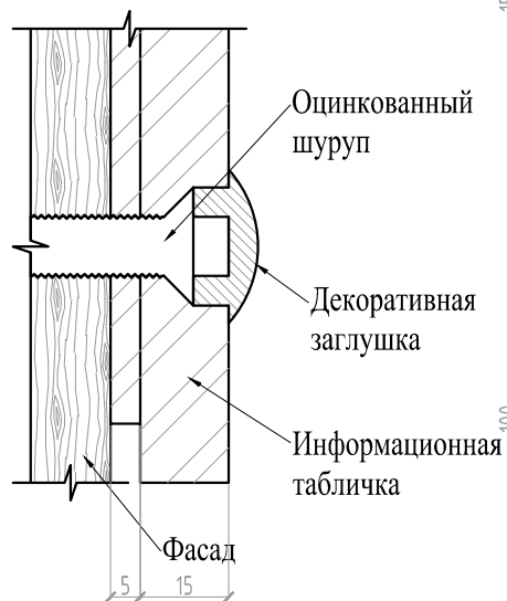
Сечение узла крепления
